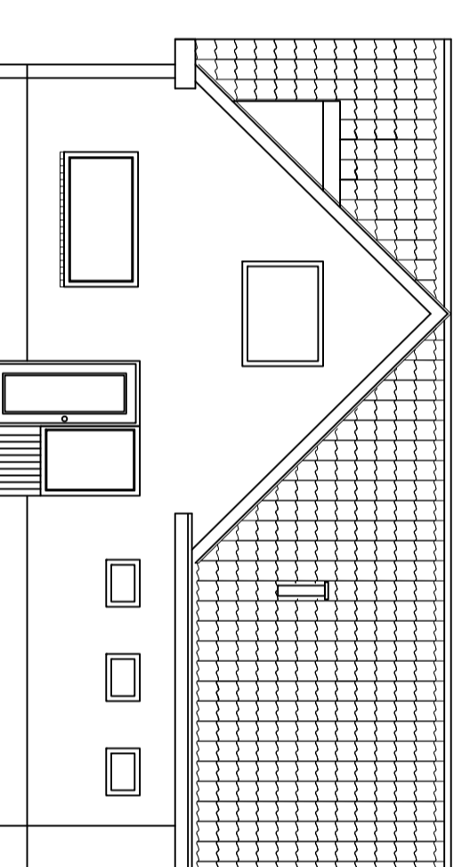
Westgevel bestand
