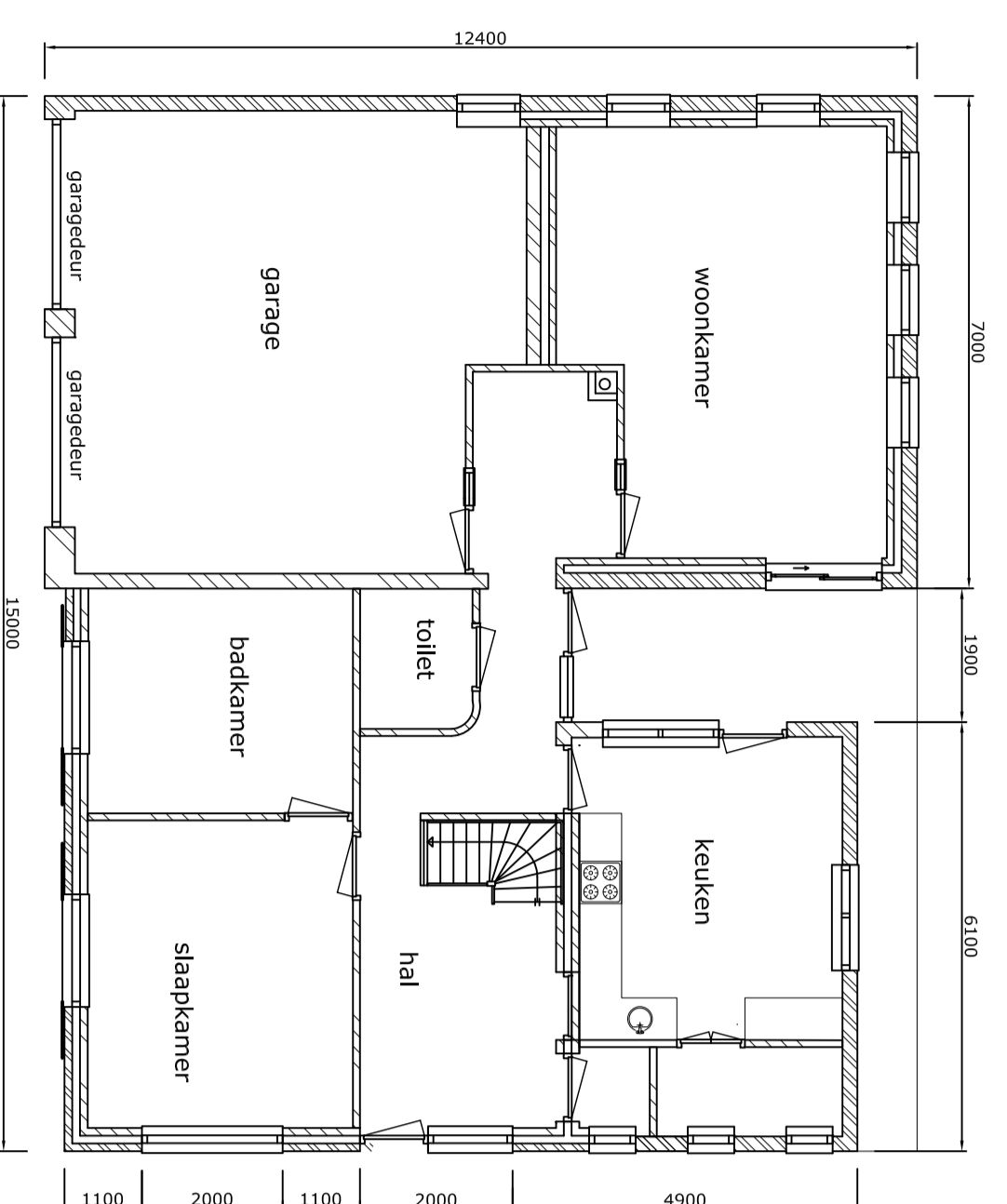
Bestaande grond bestand
